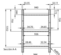
Sección A-A
