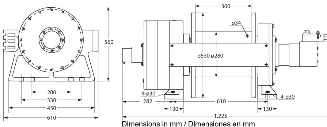
Dimensions in mm / Dimensiones en mm
